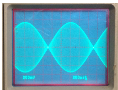
Bild 5: HF 2-Ton Signal im Zeitbereich mit einem scharfem X in den Schnittpunkten
