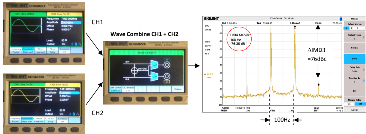
Bild 4: IMD3-Messung über die "Wave-Combine" Funktion, f1=7,050MHz, f2=7,0501MHz, Pe=2x0dBm
