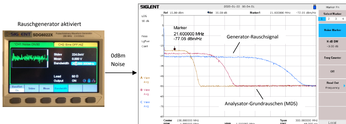
Bild 7: Rauschsignal mit 0dBm Leistung, bezogen auf 0-50MHz, 100MHz und 200MHz
