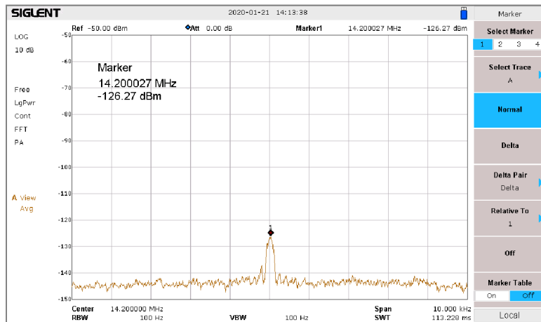
Bild 11: Erzeugung eines -126dBm-Signals mit gewählter 126dB Dämpfung, f=14,2\text{MHz}
