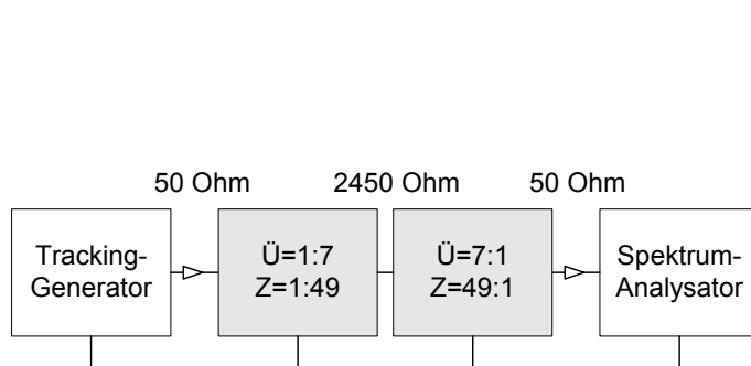
Messaufbau zur Ermittlung der Durchgangsdämpfung des Übertragers
