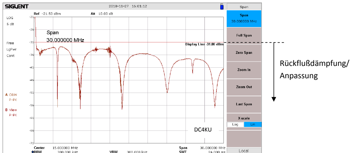
Bild 2: Typische Rückflußdämpfung einer 5-Band HyEndFed-Antenne, SWR \leq 1,2 auf Resonanzen
