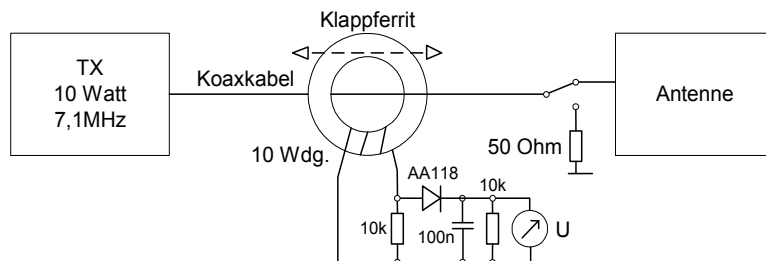
Bild 3: Einfache HF-Stromzange als Indikator von Mantelstrom auf Leitungen
