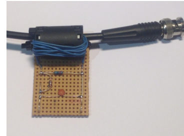
Bild 3: Einfache HF-Stromzange als Indikator von Mantelstrom auf Leitungen
